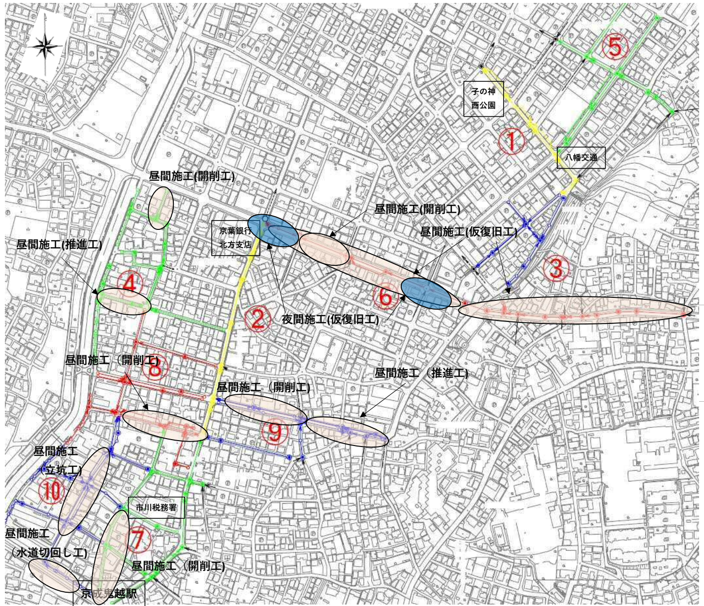
平 面 図
